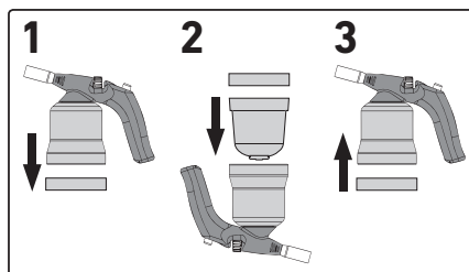
Obr. 4, vloženie kartuše
